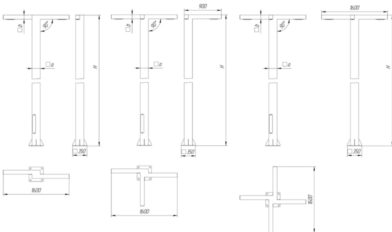
VL-FLAT 30x2
